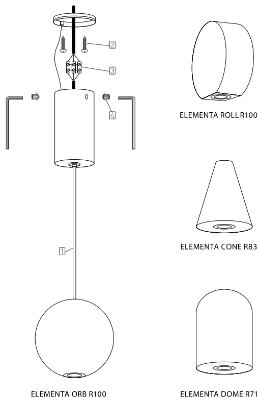
Рис. 1. Установка и подключение светильника
