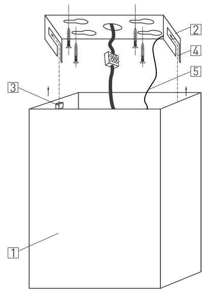
Рис. 2. Установка и подключение светильника
